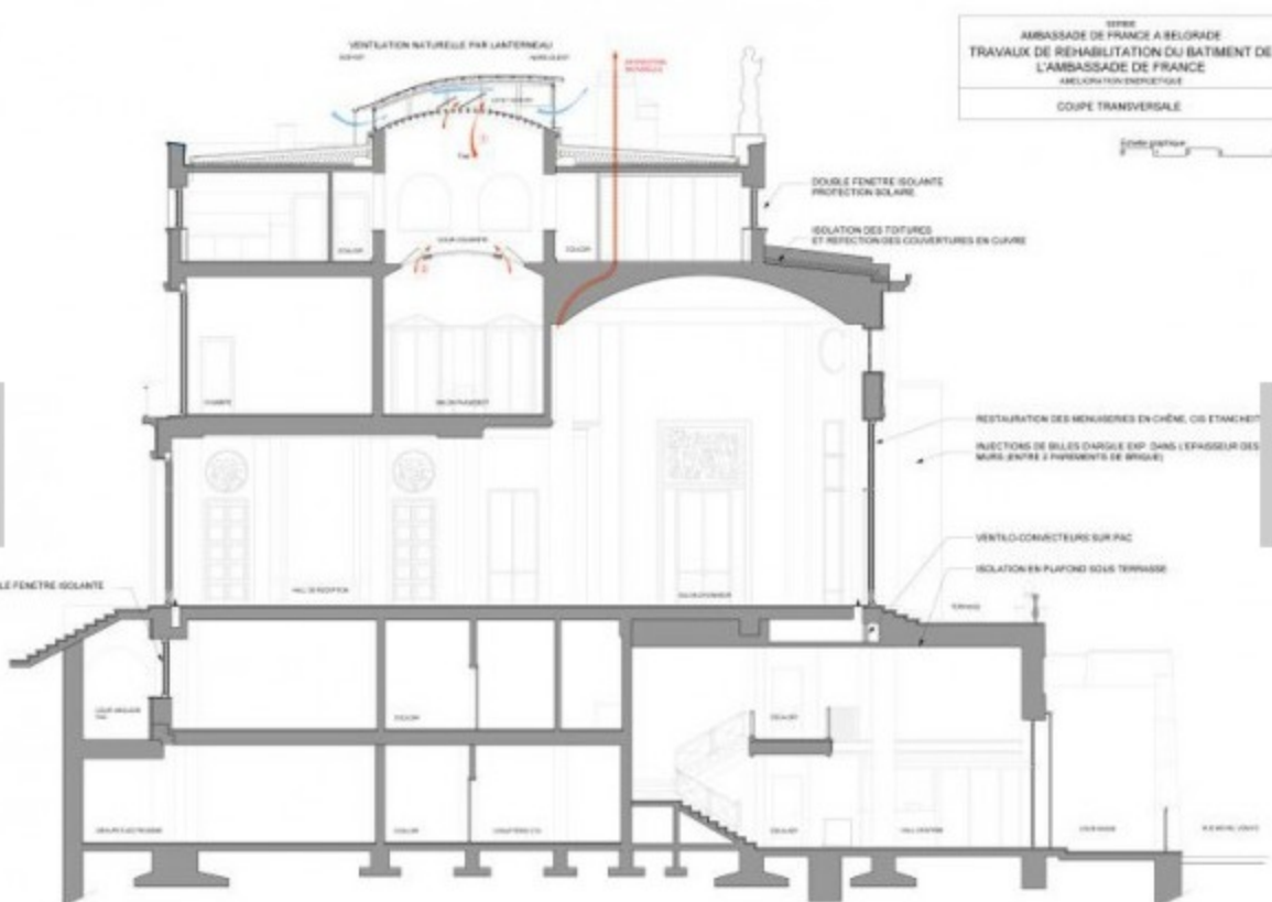
Ambassade de France en Serbie, coupe transversale © ARC&SITES
